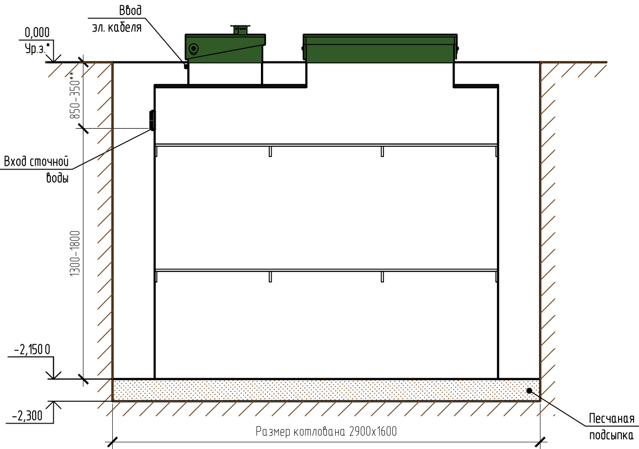
Вид А
