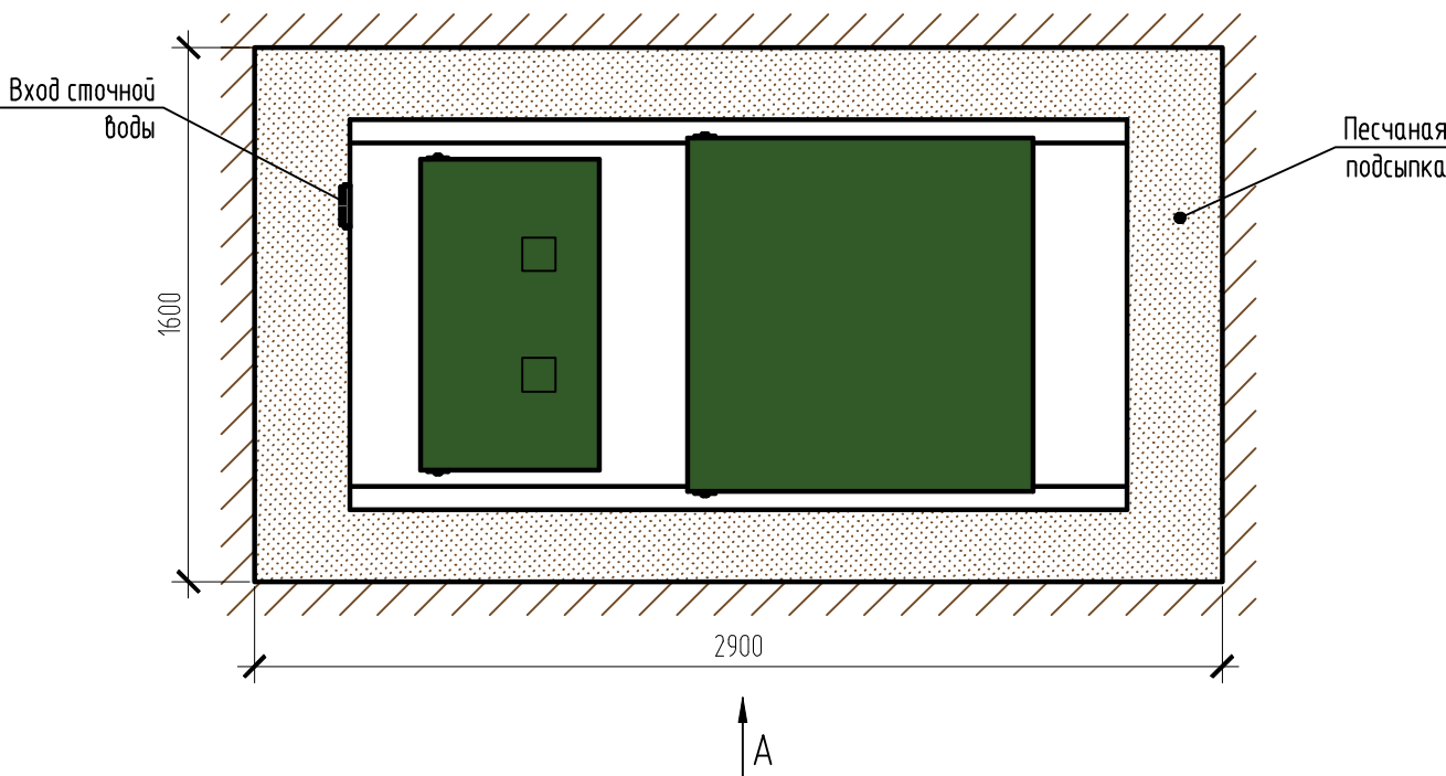
Вид сверху
